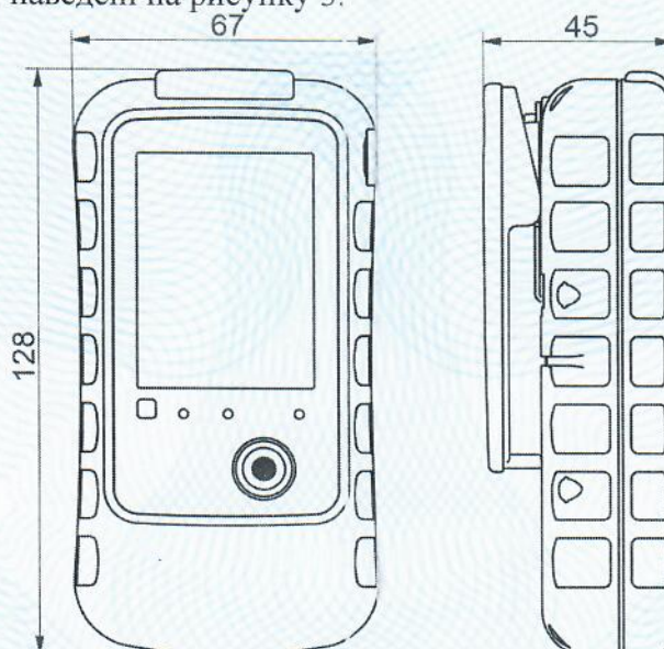
Рисунок 3 – Габаритні розміри приладу.
